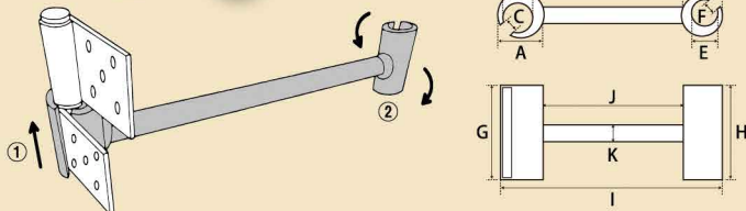
各部寸法
